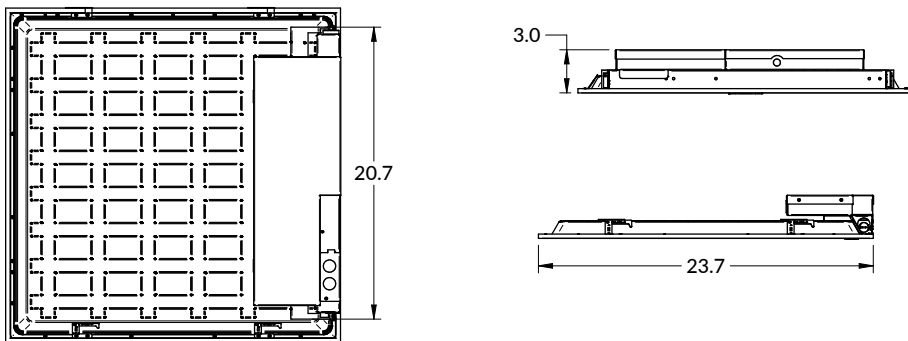
2x2 VPAN-CR-EM10
