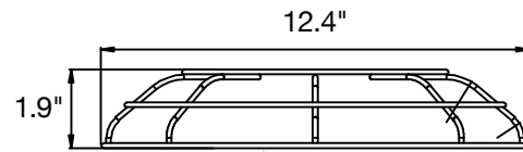
Acrylic Reflector (90°) RHB-240-ACR-RF
