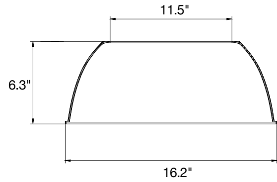
Acrylic Reflector (90°) RHB-240-ACR-RF
