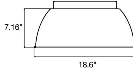
Aluminum Reflector RHB3-240-ALM-RF-90
